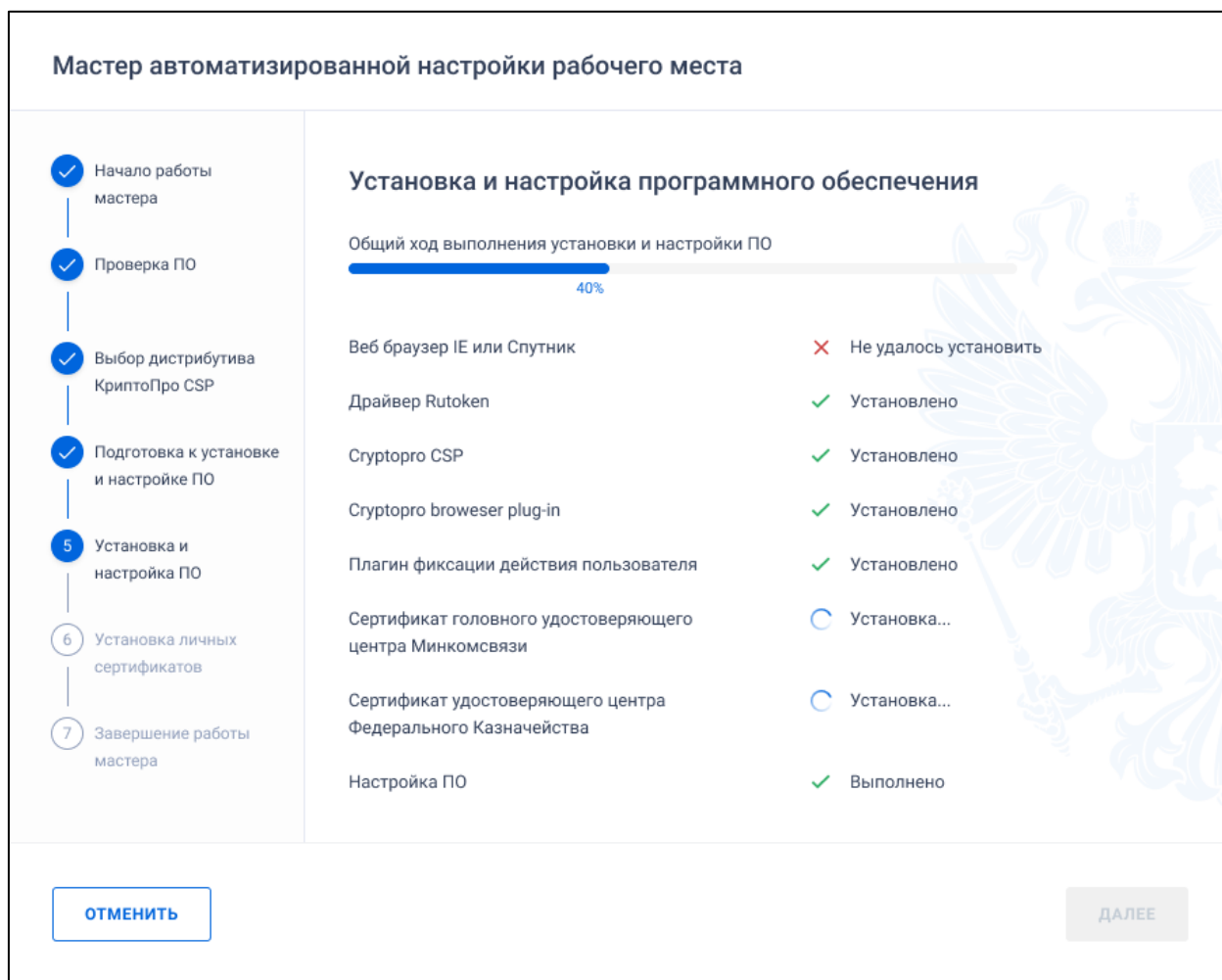
Рисунок 7. Окно установки компонентов и настройки приложений
