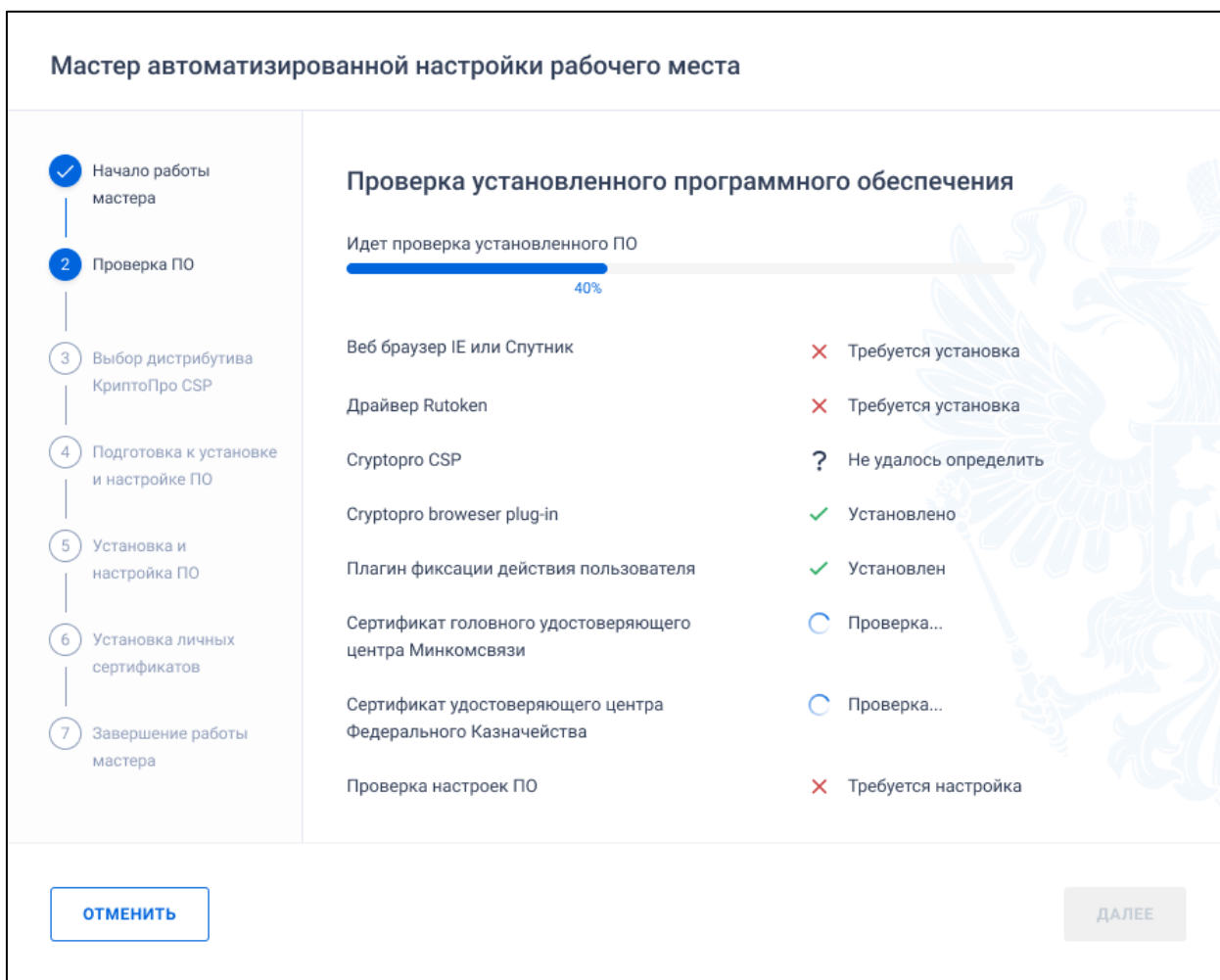
Рисунок 11. Окно проверки установленного программного обеспечения на ОС Linux
