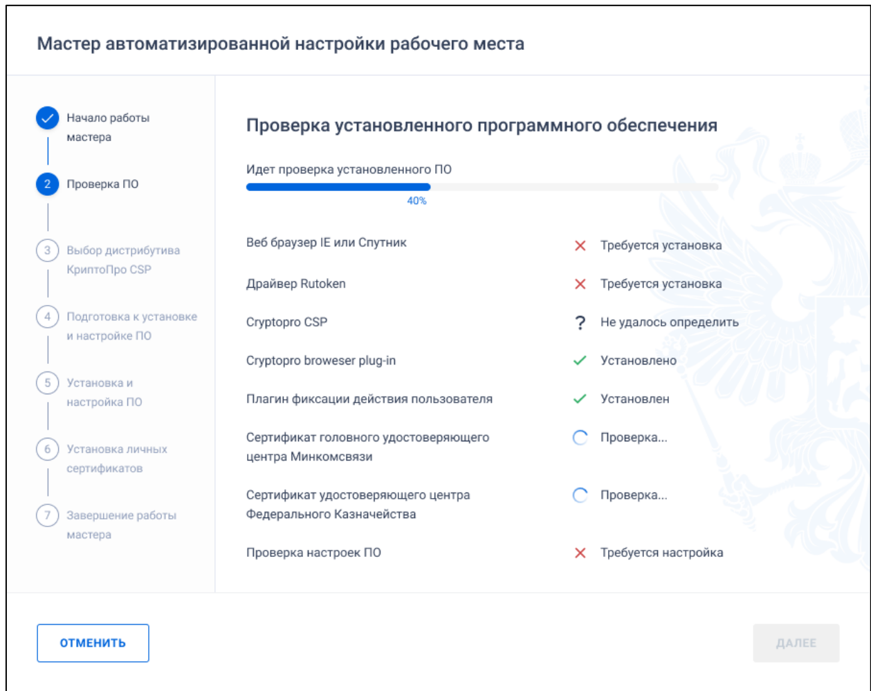
Рисунок 3. Окно проверки установленного программного обеспечения
